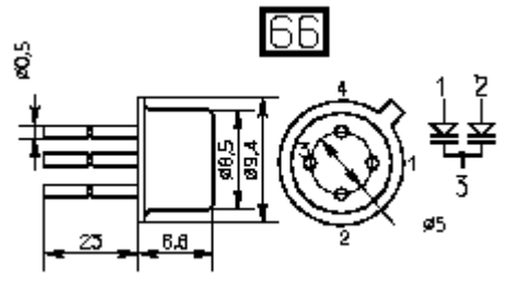
2В118
