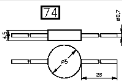
2С101
