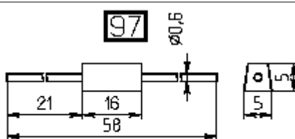
КД257, КД258
