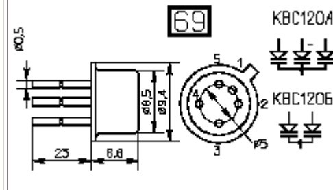
КВС120
