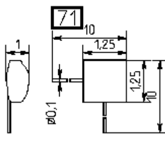
КВ116, КВ140-1
